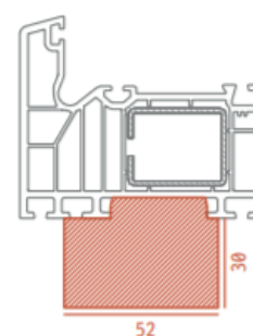
U=0,74 W/m 2 K Schüco SI 82, Alu Inside
